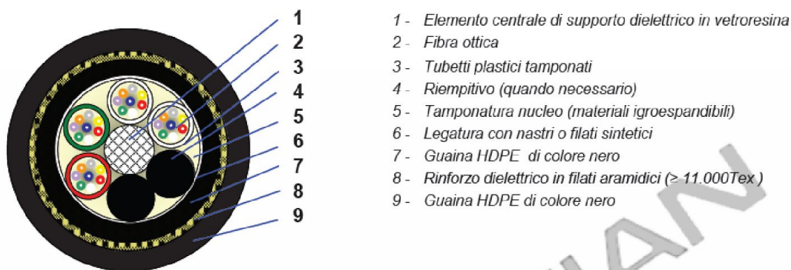
Figura 9 - Sezione di cavo autoportante a 48 fibre ottiche SMR per posa su palificata
