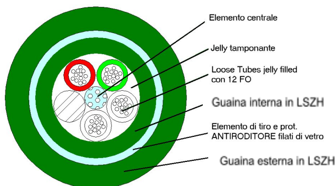
Figura 4 - Sezione di cavo a 48 fibre ottiche SMR (un tubetto riempitivo) e 24 fibre
