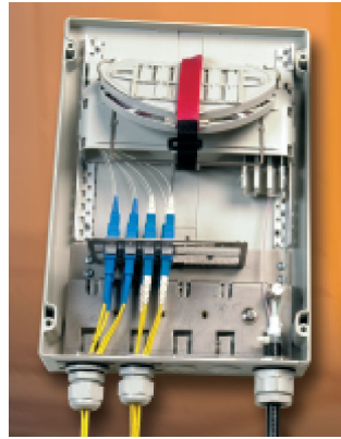
Figura 11 – Esempio di borchia a 8 terminazioni
